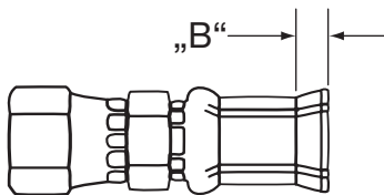
Aspetto delle serie di raccordi 91N dopo la pressatura
