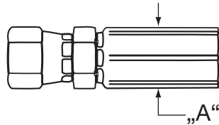
Aspetto delle serie di raccordi 56 e 93N dopo la pressatura
